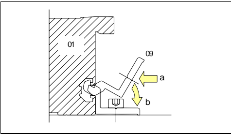
Abb.29 Klemmhalter in rechtes Kollektorprofil einhaken
