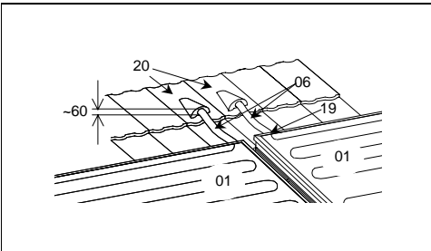
Abb.38 Detailansicht Kollektorfeldanschluss
