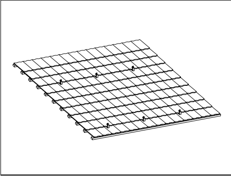
Abb.10 Dachhaut mit Dachankern
