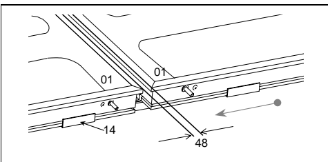
Abb.32 Zweiten Kollektor ausrichten
