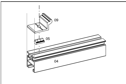
Abb.27 Einsetzen der Nutsteine für Klemmhalter
