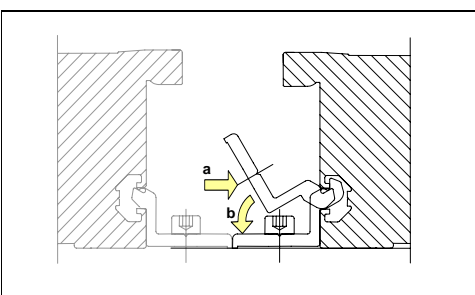
Abb.33 Klemmhalter in Basisprofil einhaken
