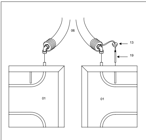
Abb.36 Anschluss des Temperaturfühlers
