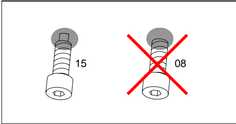
Abb.21 Stanzschraube / Zylinderkopfschraube
