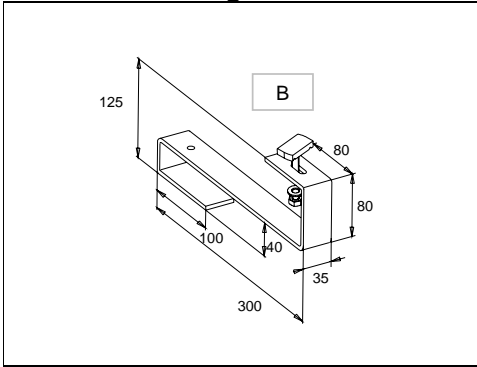
Abb.7 Maße Dachanker B
