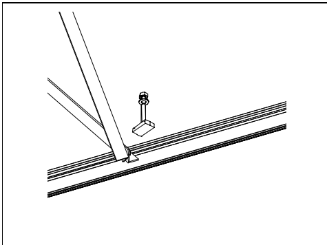
Abb. 16 Befestigung mit Formschluss-Schraube
