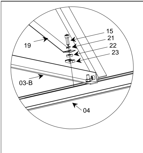
Abb.22 Befestigung Sicherungskreuz-Basisprofil
