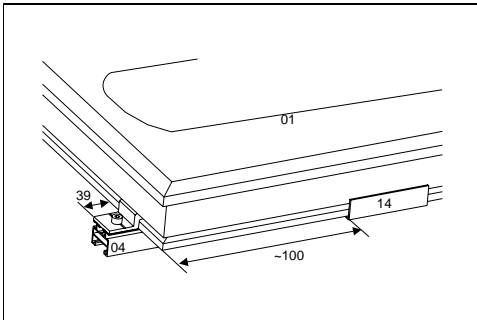
Abb.26 Ausrichten des ersten Kollektors
