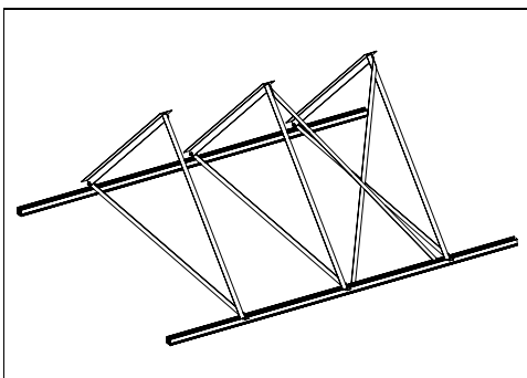
Abb.23 Befestigung der weiteren FD-Montagewinkel
