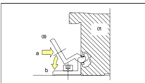
Abb.28 Klemmhalter in linkes Kollektorprofil einhängen
