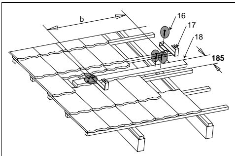
Abb.9 Befestigung Montagebrett und Dachanker
