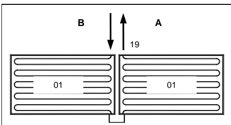
Abb.35 Kollektorfeldanschluss
