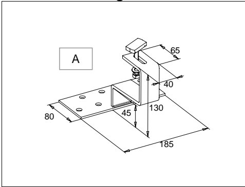
Abb.4 Maße Dachanker A
