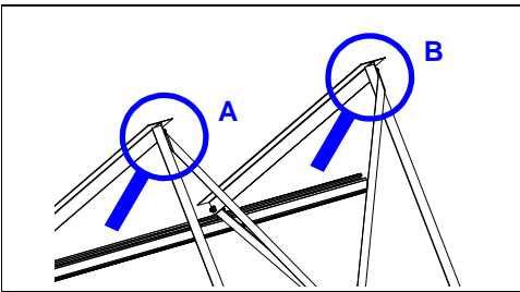
Abb.19 Detailansicht Sicherungskreuz
