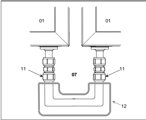
Abb.34 Hydraulische Verbindung
