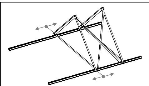
Abb.20 Befestigung des zweiten FD-Montagewinkels
