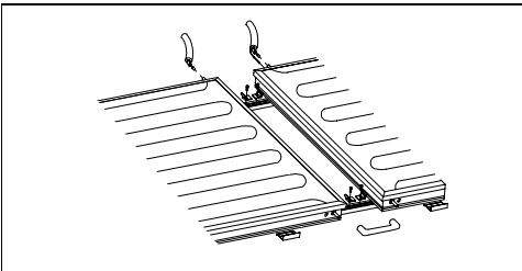
Abb.31 Zweiten Kollektor aufbringen
