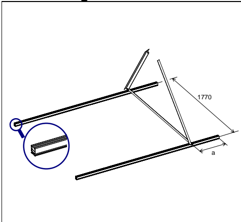
Abb. 15 Montage des ersten FD-Montagewinkels
