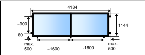
Abb.2 Aufdach-Montage-Set2
