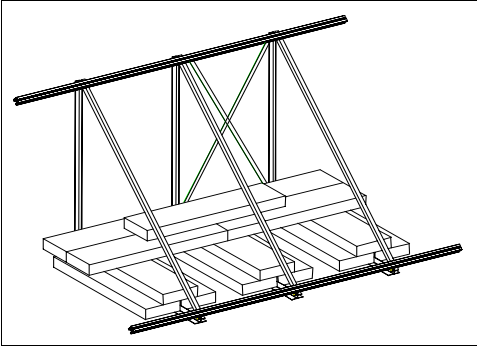
Abb.24 Standsicherheit (Beschwerung)
