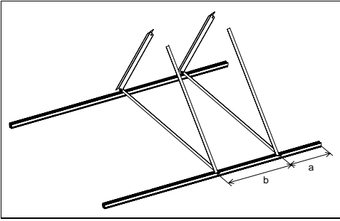
Abb.17 Zweiten FD-Montagewinkel montieren
