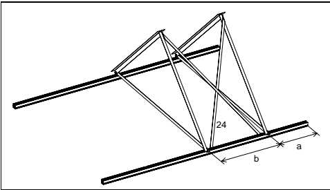
Abb.18 Sicherungskreuz montieren
