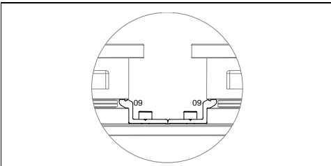
Abb.30 Nutstein ausrichten für weiteren Klemmhalter
