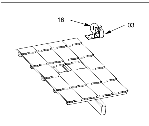
Abb.6 Montage des Dachankers A
