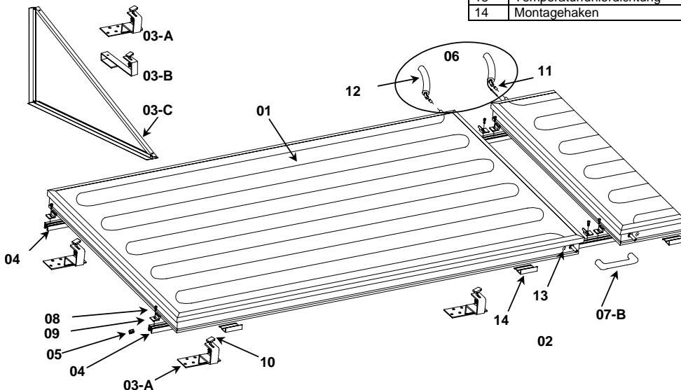
Abb. 1 Montageübersicht, waagerechte Kollektorausrichtung
