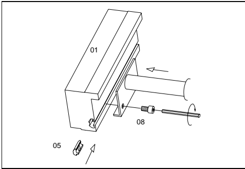
Abb.25 Befestigung der Tragegriffe
