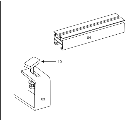
Abb.11 Befestigung des Basisprofils
