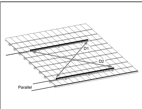
Abb.12 Ausrichten der Basisprofile
